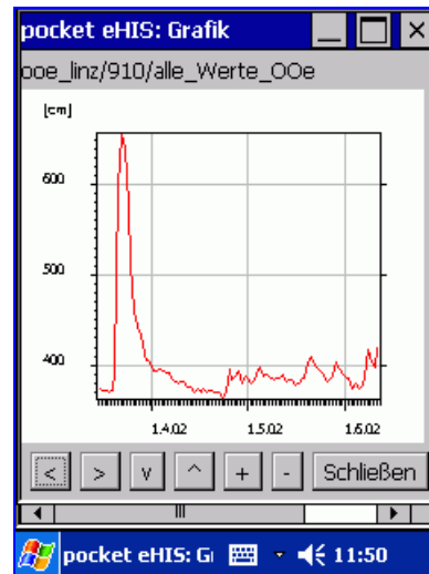
Abb. 6: Wasserstandsganglinie
