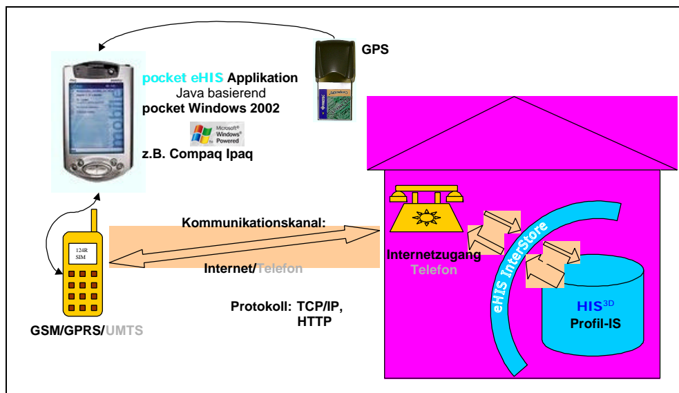
Abb. 2: Der technische Aufbau von pocket eHIS
