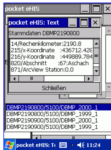
Abb. 4: Stammdatenabfrage
